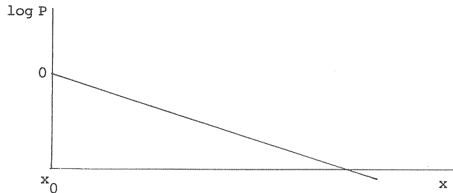
Fig. 12.1. Verdeling van hoogwaterstanden in Hoek van Holland.
