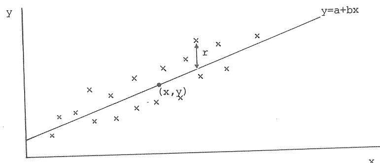
Fig. 12.2. Lineaire regressie van y op x.
