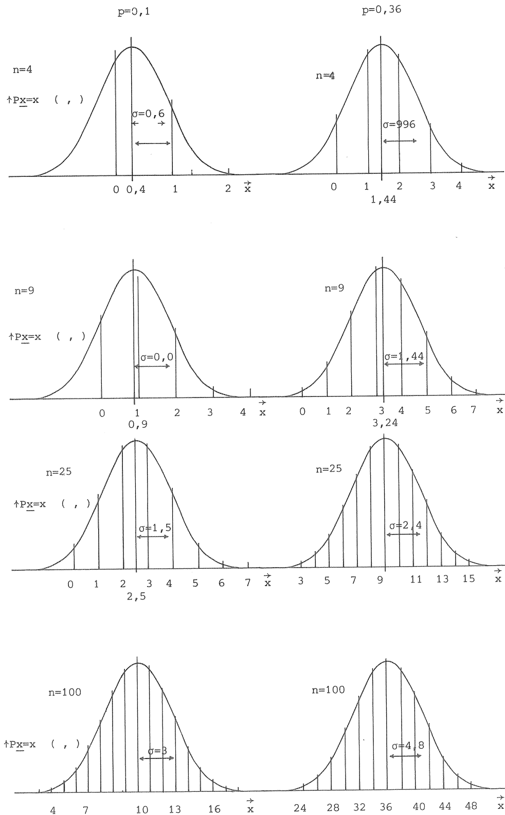
FIG 11.1. Convergentie van de binomiale verdeling naar de normale.
