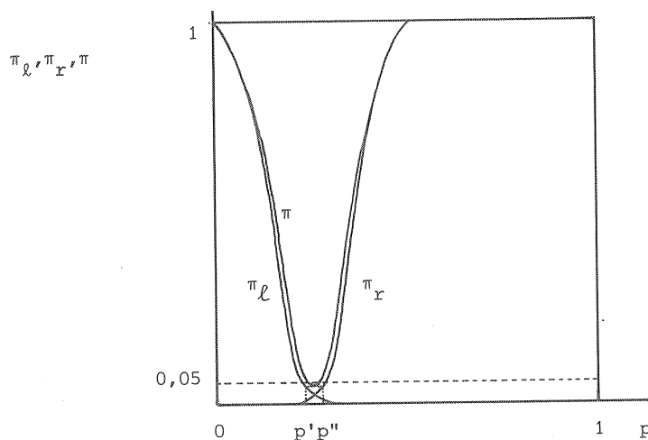
Fig.13.1. Het onderscheidingsvermogen van de binomiale toets met n = 50 , Z_{\ell}: x \leq 6 en Z_r: x \geq 19 .
