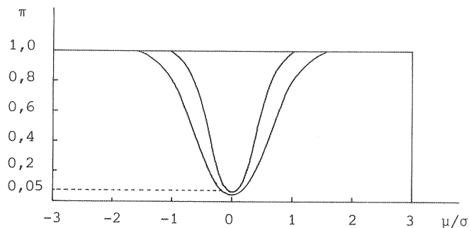
Fig. 14.4.2. Onderscheidingsvermogen van de tekentoets in vergelijking met de toets van Student (één steekproef, \alpha = 0,05 tweezijdig, n = 20 ).
