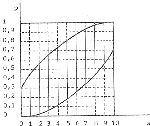
Fig. 15.1. Betrouwbaarheidsintervallen voor p bij n = 10 en \alpha_L = \alpha_R = 0,025 .
