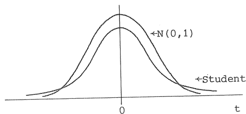
Fig. 14.2.1. Student-verdeling in vergelijking met N(0,1) .
