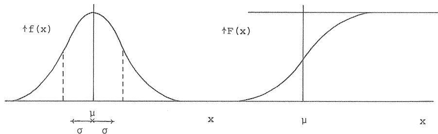
Fig. 7.1. Normale verdeling.
