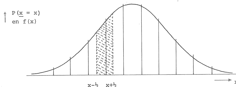
Fig. 13.2. Normale benadering van een binomiale verdeling met continuïteitscorrectie.
