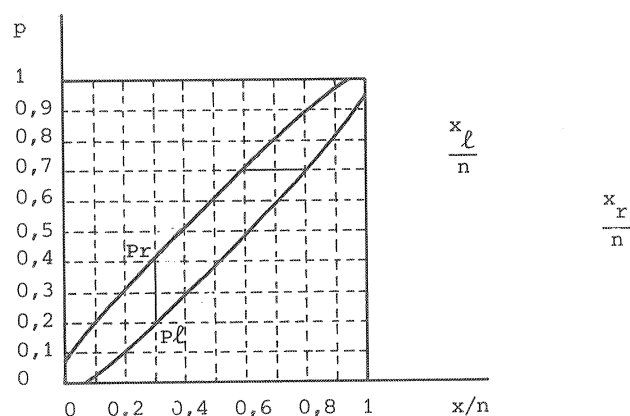
Fig. 15.2. Benaderde betrouwbaarheidsintervallen voor p
